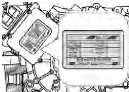
后驱动电机铭牌①打刻在后驱动电机端盖上。
